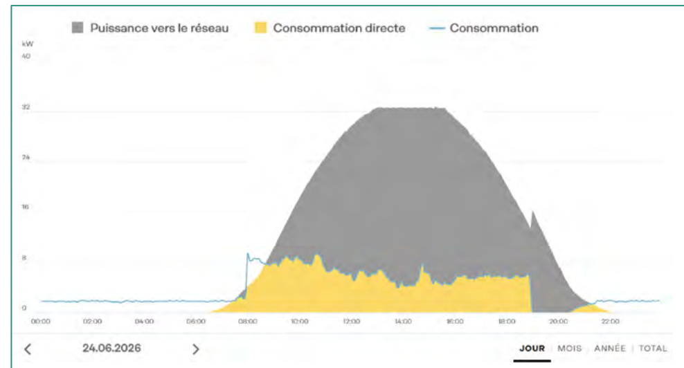
Installation photovoltaïque École de Guéthary
